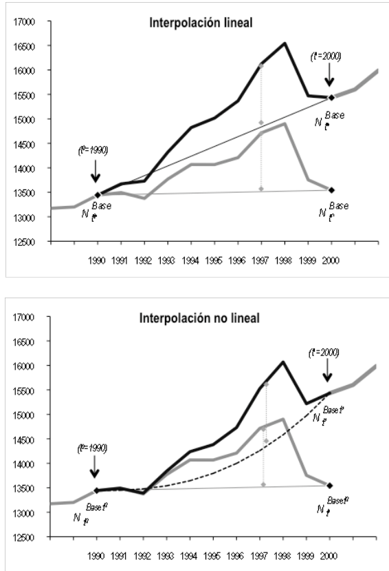
Gráfico 1. Enfoque geométrico. Método de interpolación de los valores nominales
